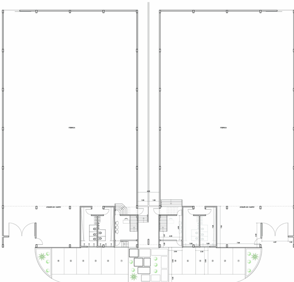
PLANTA TÉRREO esca 1: 100
